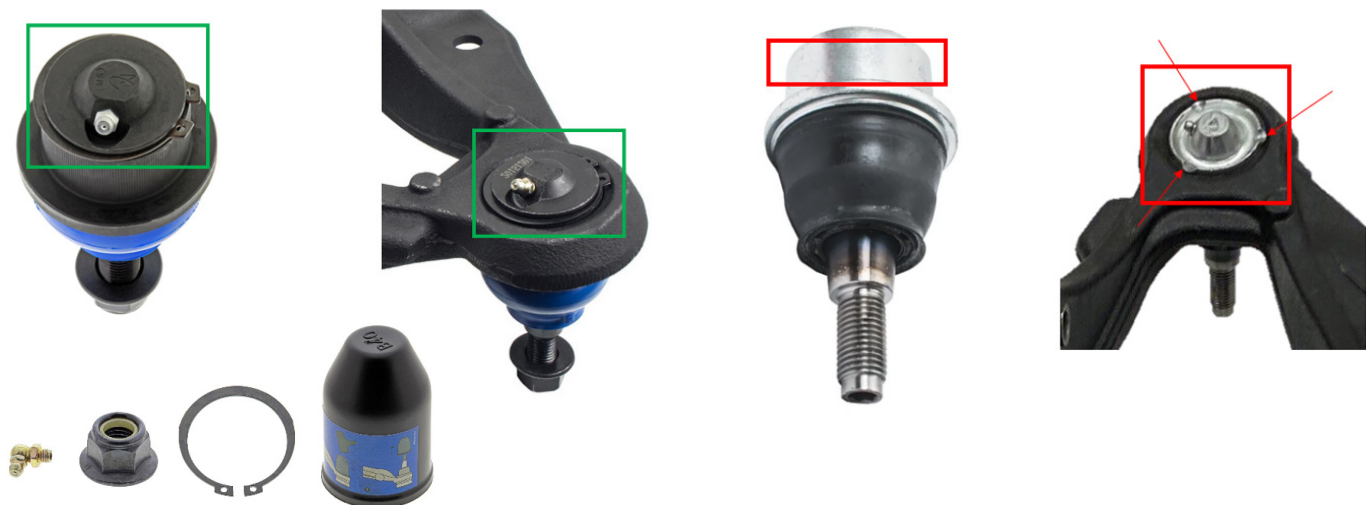
Figure 1. Le joint à rotule inférieur avant Mevotech Supreme MK6711 peut être fixé au bras de suspension facilement grâce au circlip (gauche) comparativement à la méthode de fixation ou de sertissage de la conception d'origine (droite)
