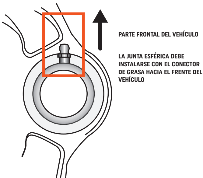
Figura 1: Orientación de instalación correcta de la junta esférica
