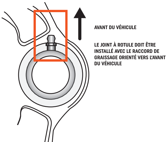
Figure 1 : Orientation d'installation adéquate du joint à rotule
