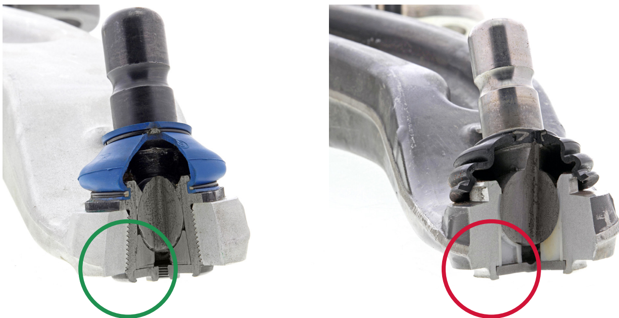
Figure 1. Palier de métal fritté basé sur la technologie bimétallique de Mevotech (gauche) par rapport à un palier de plastique d'origine (droite)
