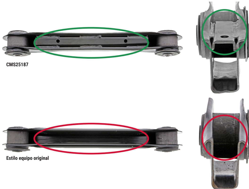
Figura 1. Brazo de control Supreme de Mevotech con perfil de estampado mejorado con refuerzo (arriba) en comparación con el brazo de control estilo equipo original (abajo)
