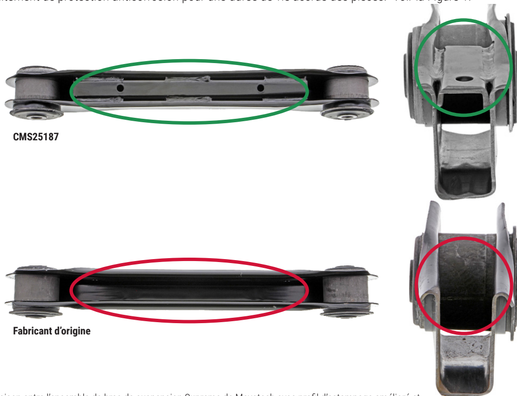
Figure 1. Comparaison entre l'ensemble de bras de suspension Supreme de Mevotech avec profil d'estampage amélioré et entretoise soudée (photo du haut) et un ensemble de bras de suspension de style fabricant d'origine (photo du bas)
