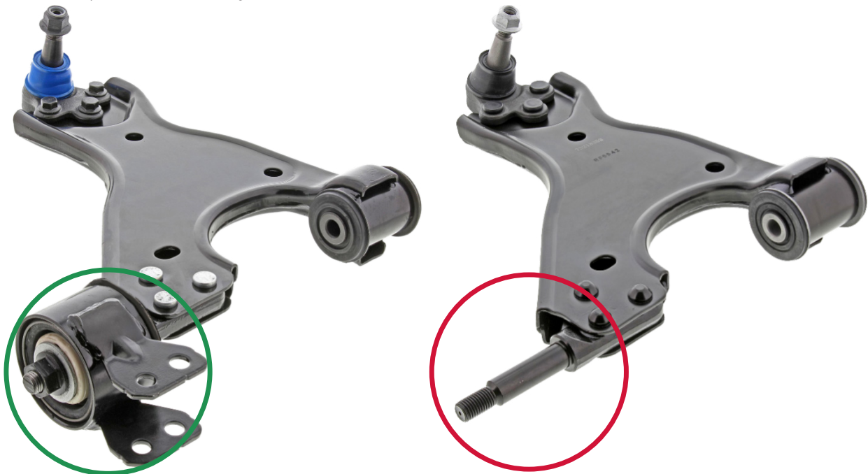
Figura 1. Conjunto del brazo de control Supreme de Mevotech con buje de conformidad preinstalado (izquierda) en comparación con el conjunto del brazo de control estilo equipo original (derecha)
