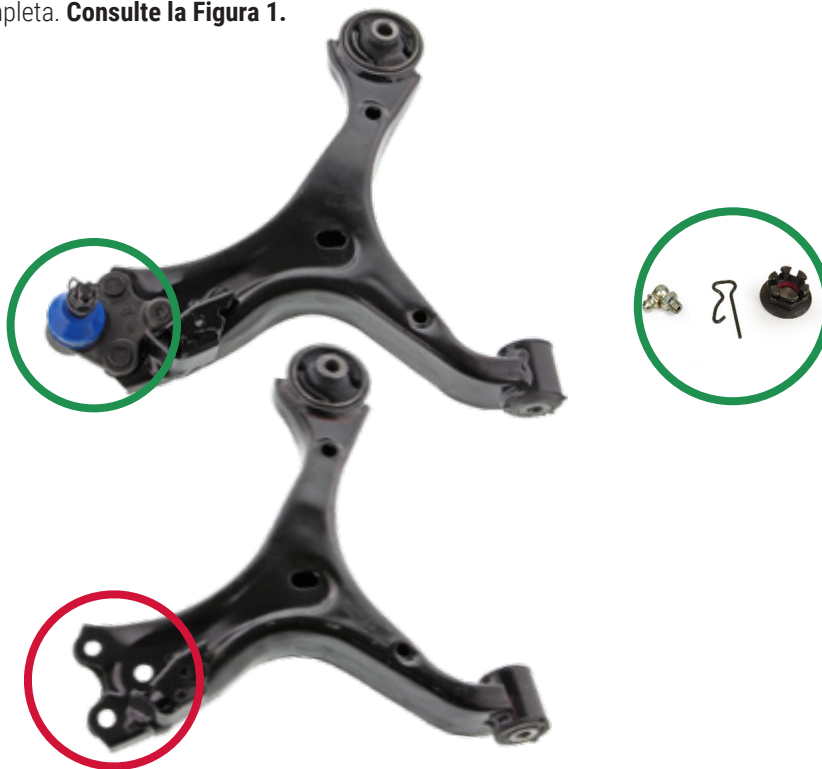
Figura 1. Conjunto del brazo de control Supreme de Mevotech con junta esférica preinstalada y hardware (arriba) vs brazo de control básico estilo equipo original (abajo)
